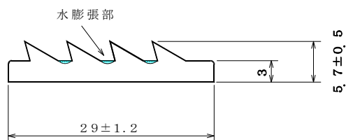
ゴム輪詳細図
