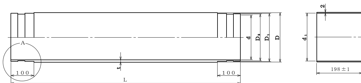
SUSカラー詳細図
