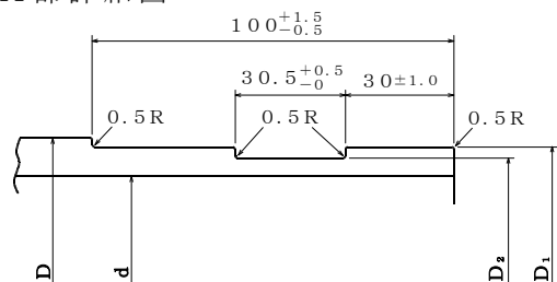
A 部詳細図
